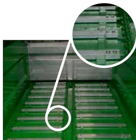
Bakbodem, bodemketting en slijtlatten
