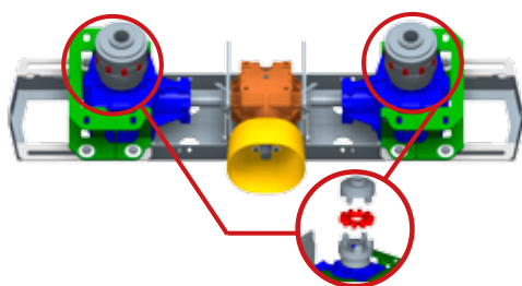
Overbrenging van de verticale strooiwalsen beschermd door elastomeer koppelingen
